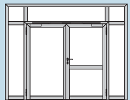
2-flg. Tür mit 2 Seitenteilen und Oberlicht
